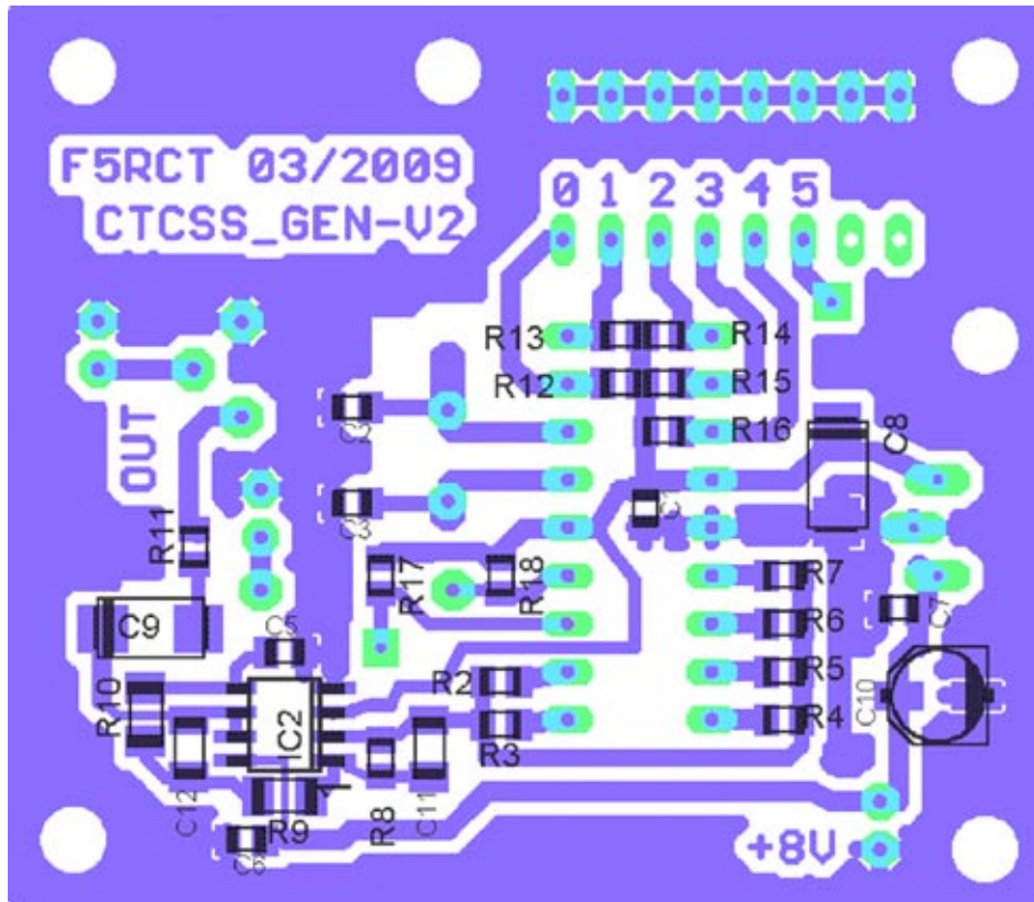
Placement des composants CMS face soudure.
