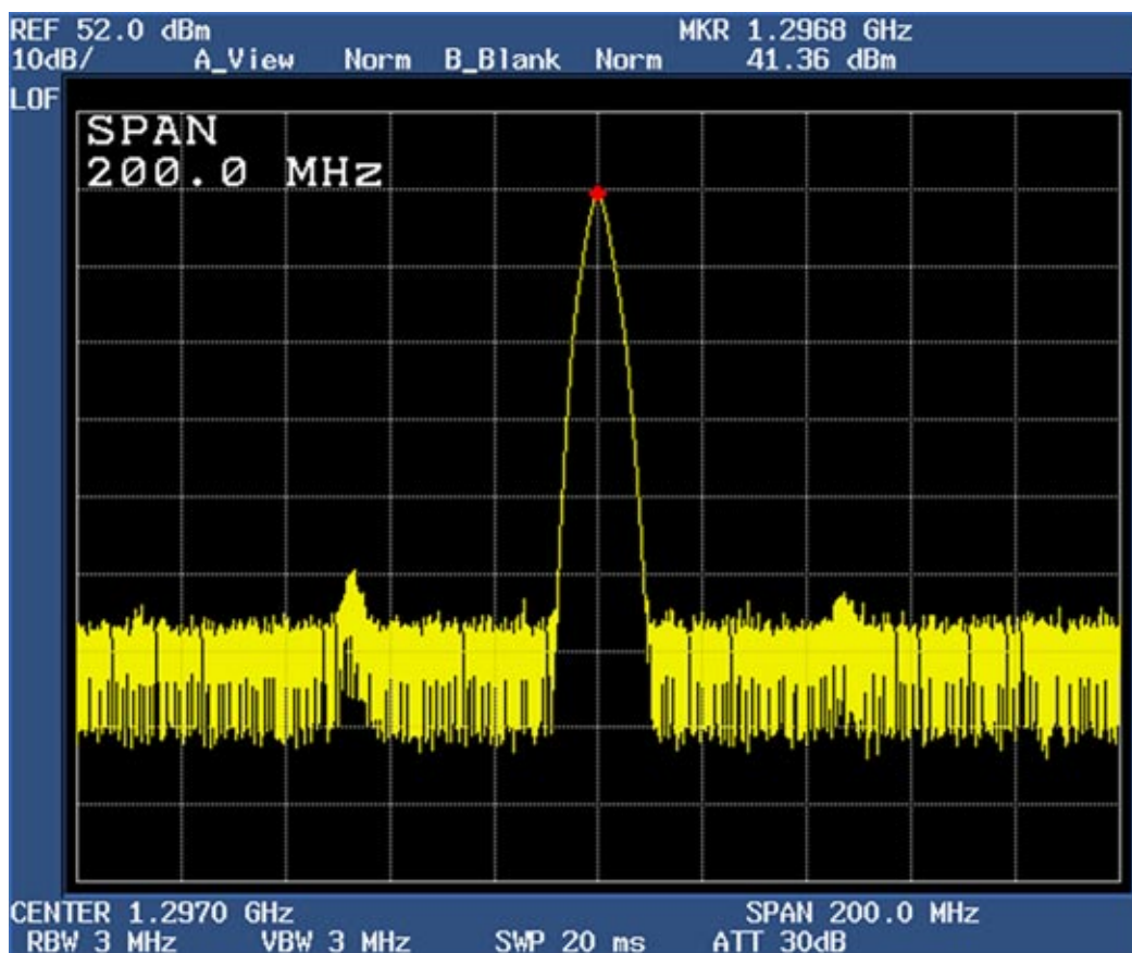
Spectre de sortie à 15W (résidus OL -50dB)
