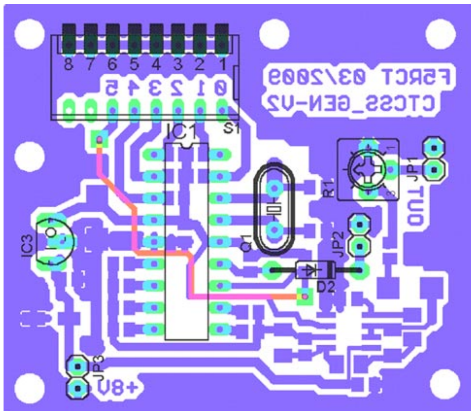
Placement des composants à souder en face supérieure.
